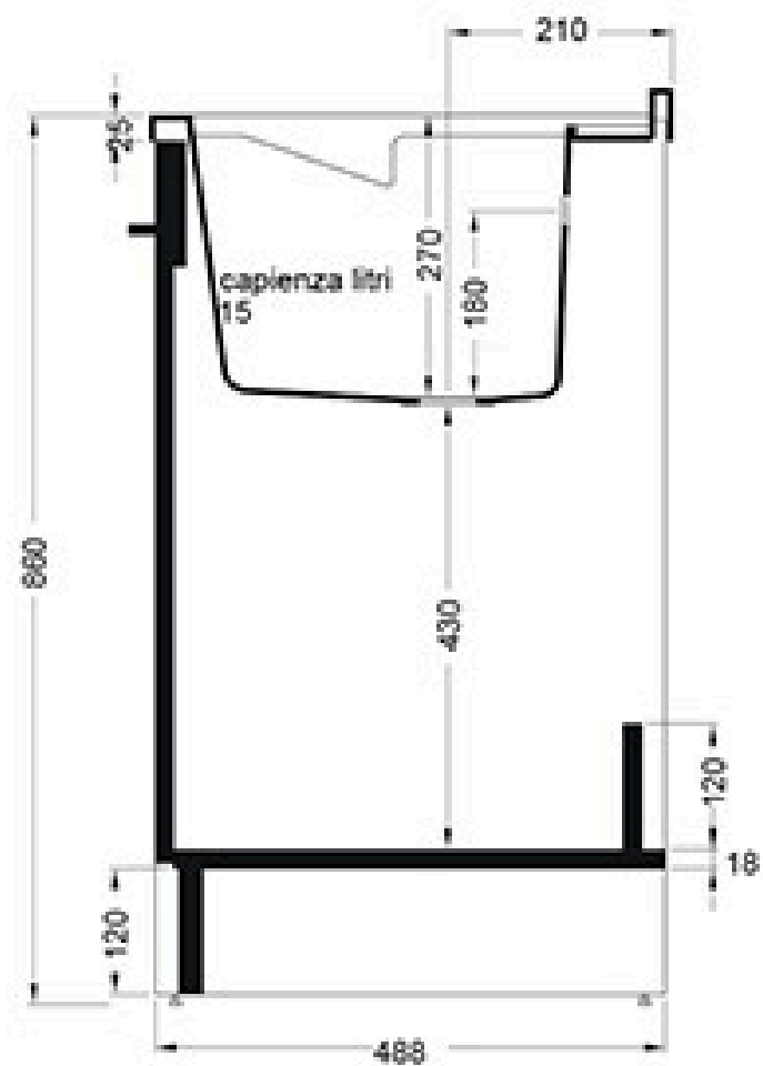
SEZIONE A-A
