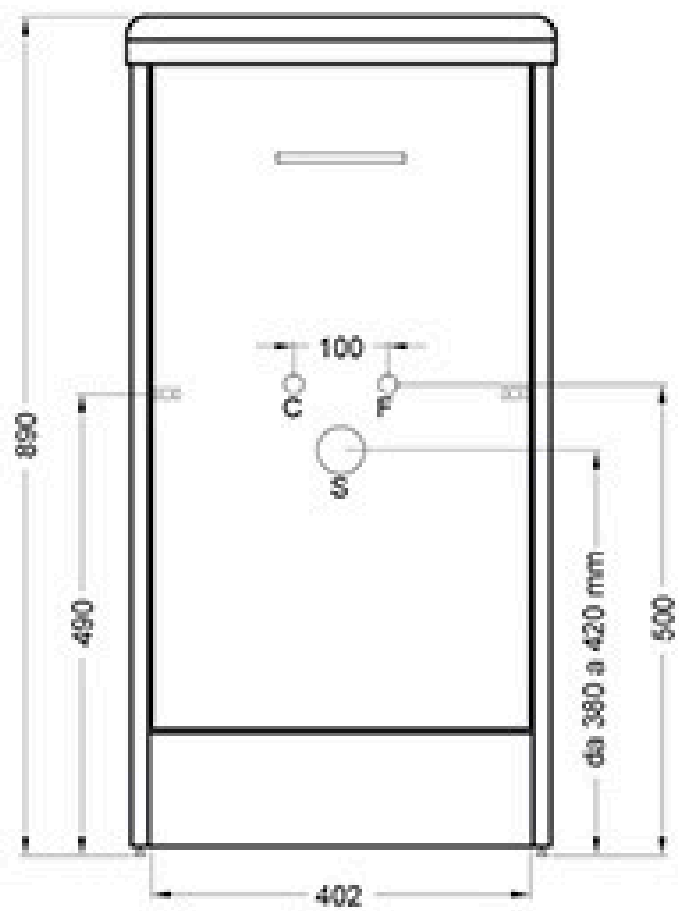
VISTA FRONTALE
